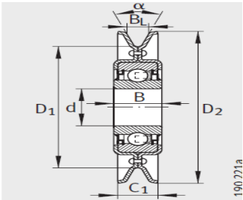
RSRA...-L0、RSRA...-KO 类型 A
