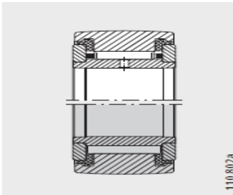
NATR..-PP (优化的 NATV..-PP INA 轮廓)
